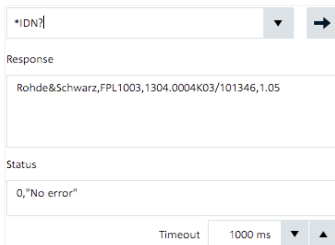
Fig. 5-23: ID String
