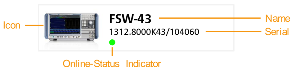
Fig. 5-3 Instrument Item
