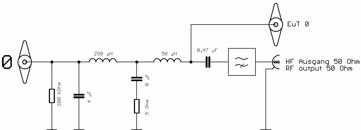
Abb. 1 Schaltplan NNLK 8122
