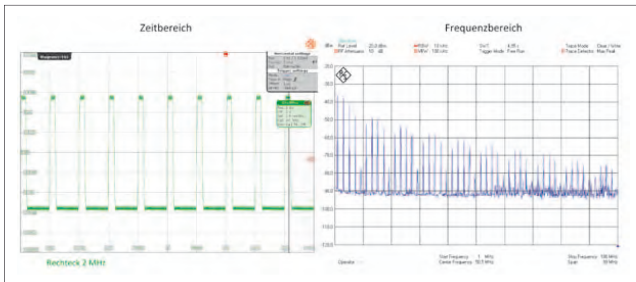
Bild 1.5 Rechteckimpuls, Darstellung im Zeit- und Frequenzbereich
