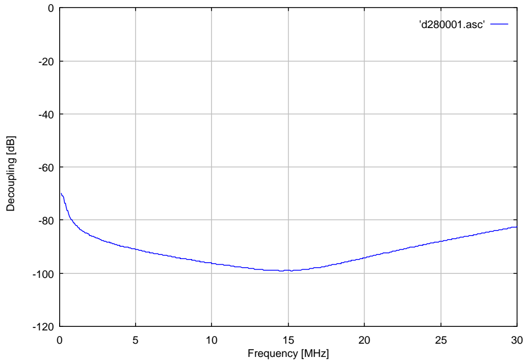
Abb. 1: Entkopplung zwischen Signalgenerator und Störquelle Fig. 1: Decoupling signal generator to interference port
