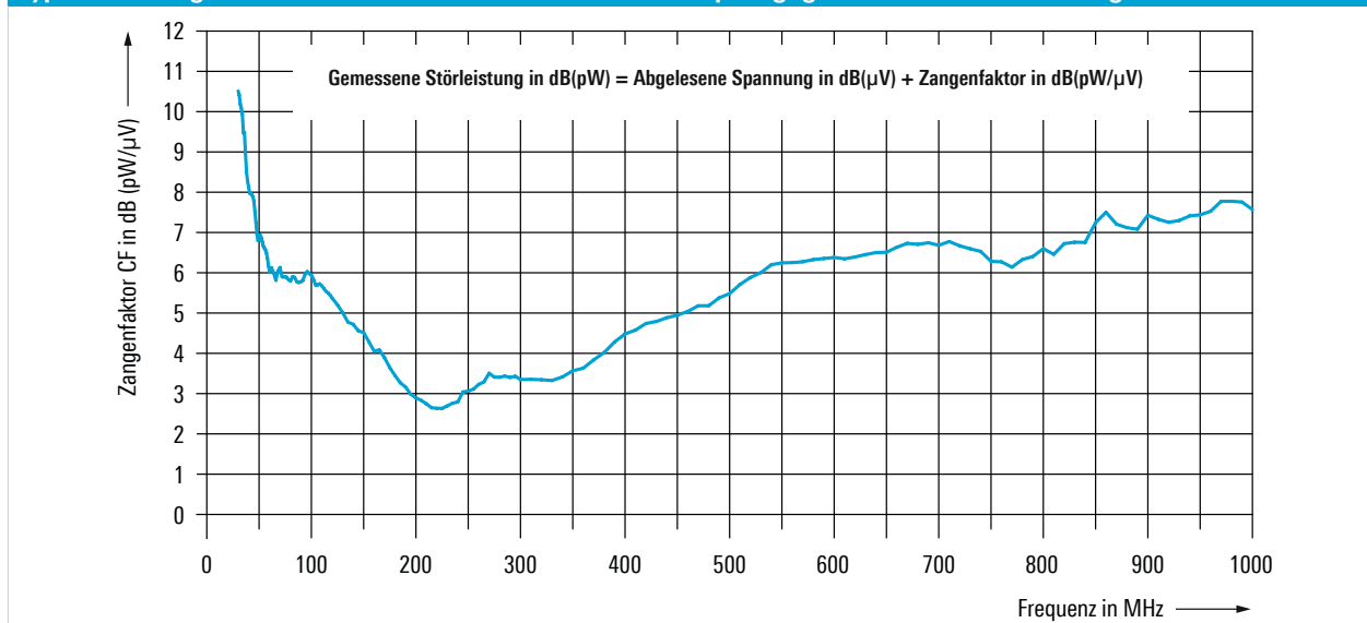
Typischer Zangenfaktor der R&S®MDS-21 mit 6-dB-Dämpfungsglied und 5-m-Verbindungskabel
