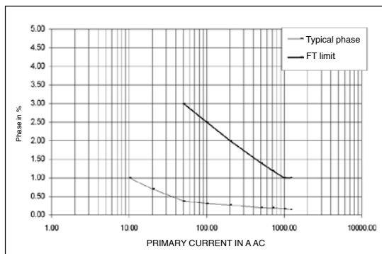
Phase shift
