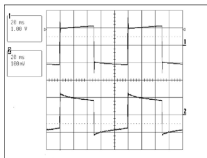
200 A calibre
