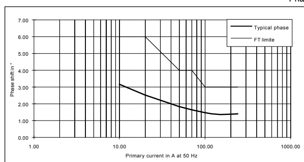
Phase shift
