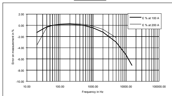
200 A calibre
