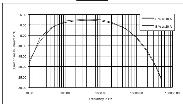
20 A calibre
