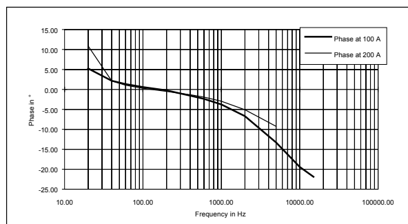
200 A calibre
