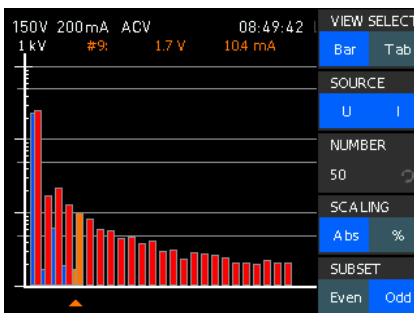
Harmonischen-Analyse: Balkendiagramm
