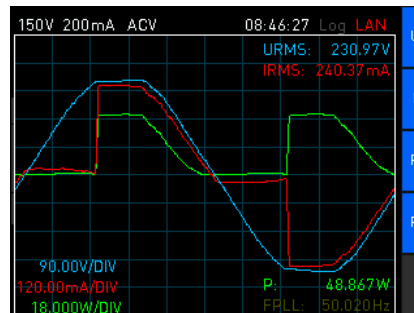
Waveform-Funktion: Verbraucher mit Phasenanschnittsteuerung
