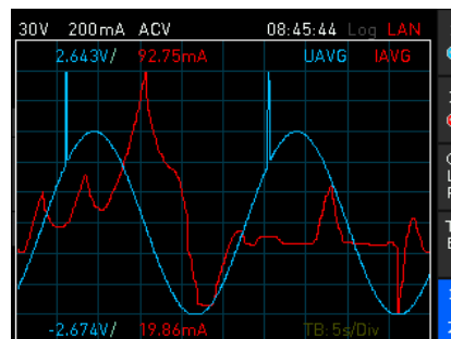
Trendchart-Funktion
