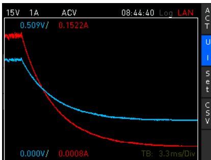
Inrush-Funktion
